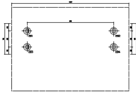
PLANTA DE LOCAÇÃO DAS ESTACAS BROCA ESCALA - 120
